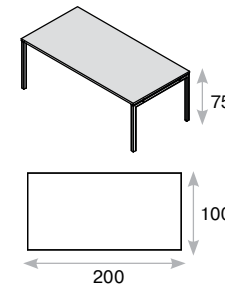
Стол для переговоров 80S065 217
